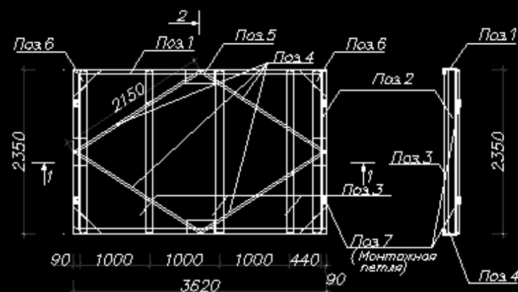
Рама Р-2
