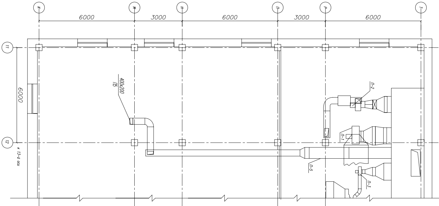
ФРАГМЕНТ ЦОКОЛЬНОГО ЭТАЖА В ОСЯХ 11-12/К-Т
