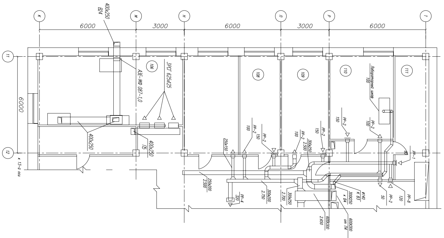
ФРАГМЕНТ ПЛАНА 1-ГО ЭТАЖА В ОСЯХ 11-12/К-Т
