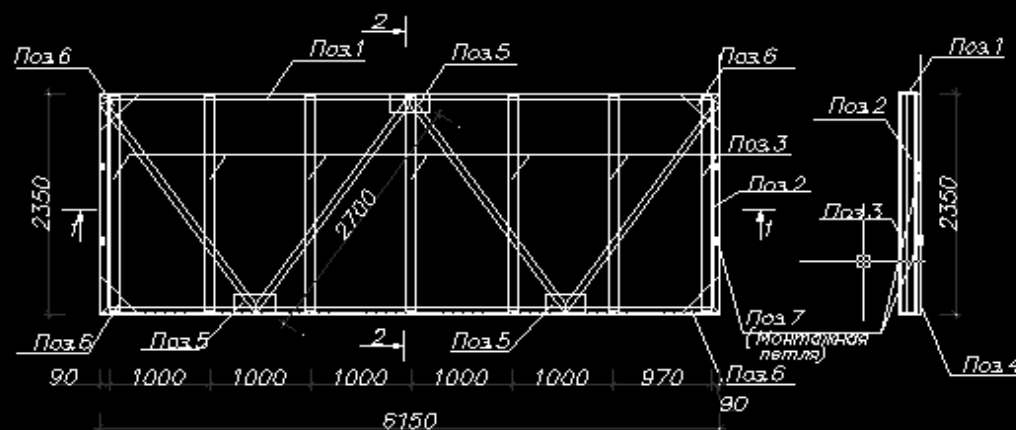
Рама Р-1
