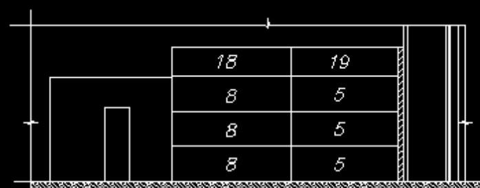
Разрез 4-4
