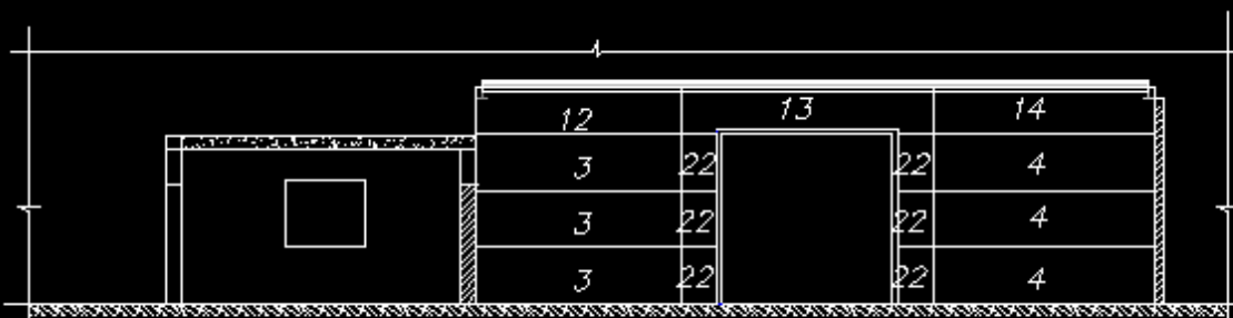
Разрез 3-3
