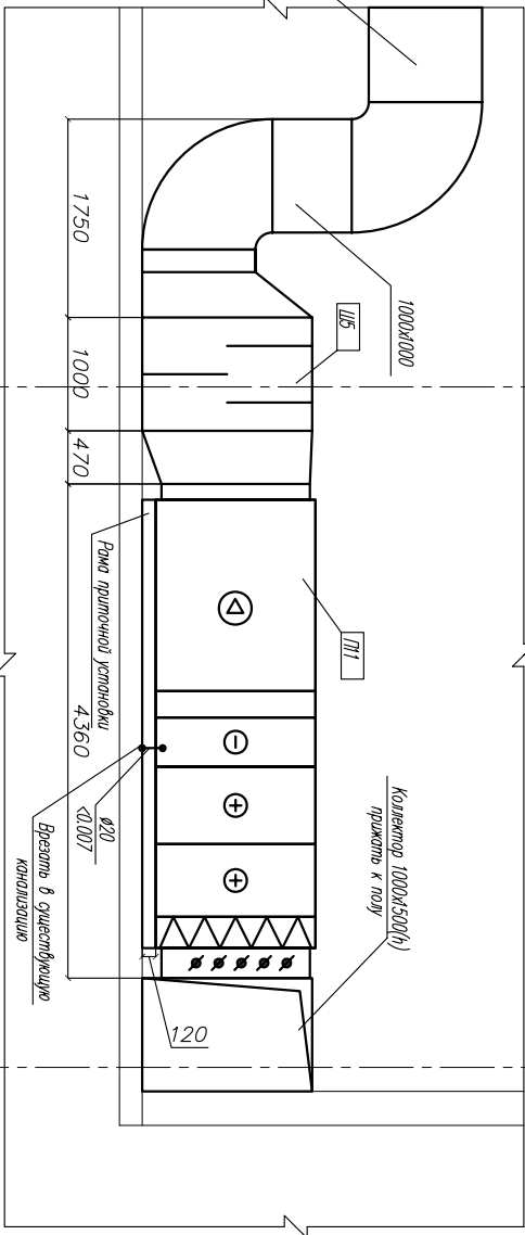
РАЗРЕЗ 2-2 М 1:50
