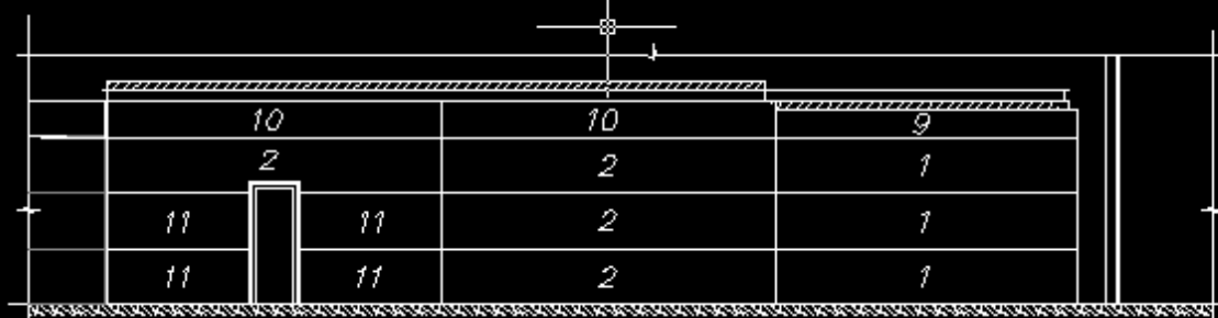
Схема расположения стеновых панелей
