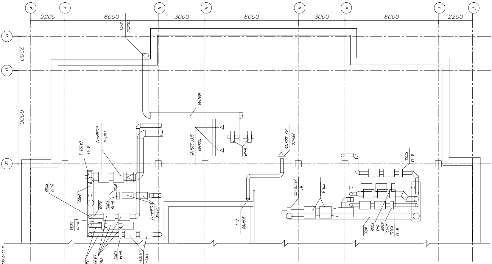
ФРАГМЕНТ ПЛАНА ТЕХНИЧЕСКОГО ЭТАЖА В ОСЯХ 11-12/К-Т
